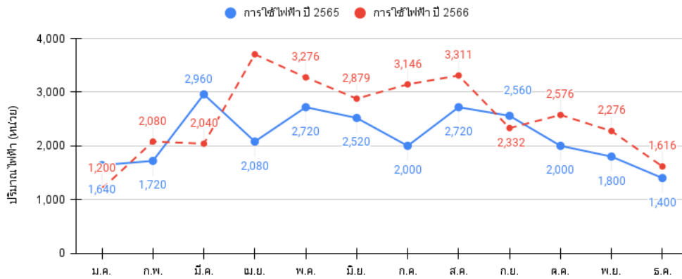
การใช้ไฟฟ้า เปรียบเทียบปี 2565-2566
